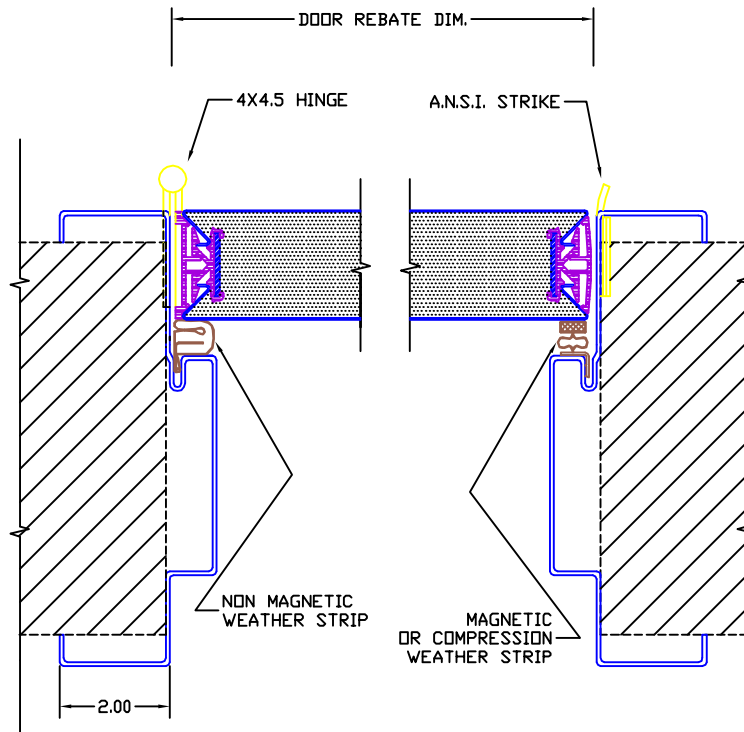
HINGE JAMB DETAIL
